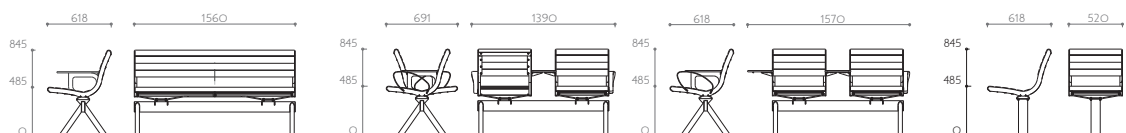
Banc 3 places Réf. 12 4530A - 67 kg
