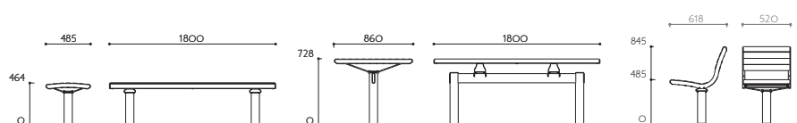
Banquette 3 places Réf. 12 4535B - 47 kg
